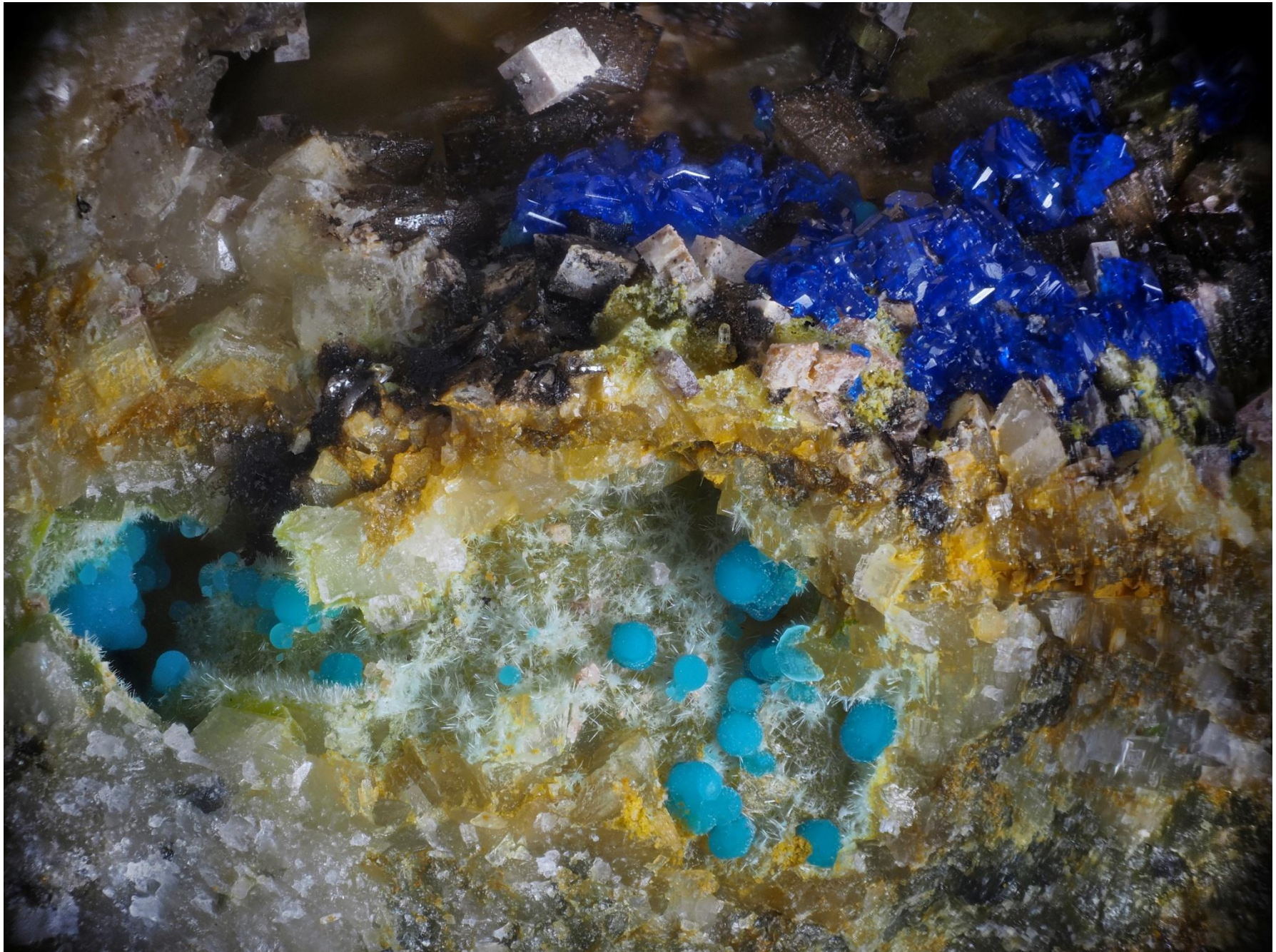
Rosasite Azurite – Bou Skour - Maroc champ 4,8 mm
